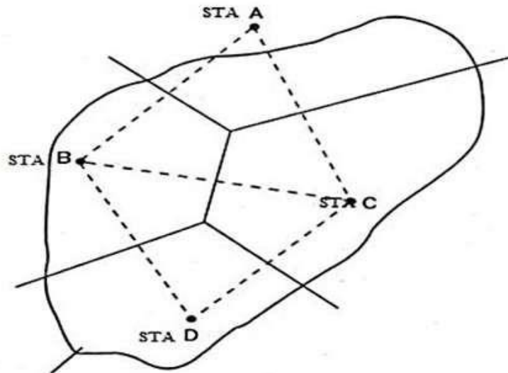
Gambar 2.11. Poligon Thiessen (Sumber : N, Djali)
