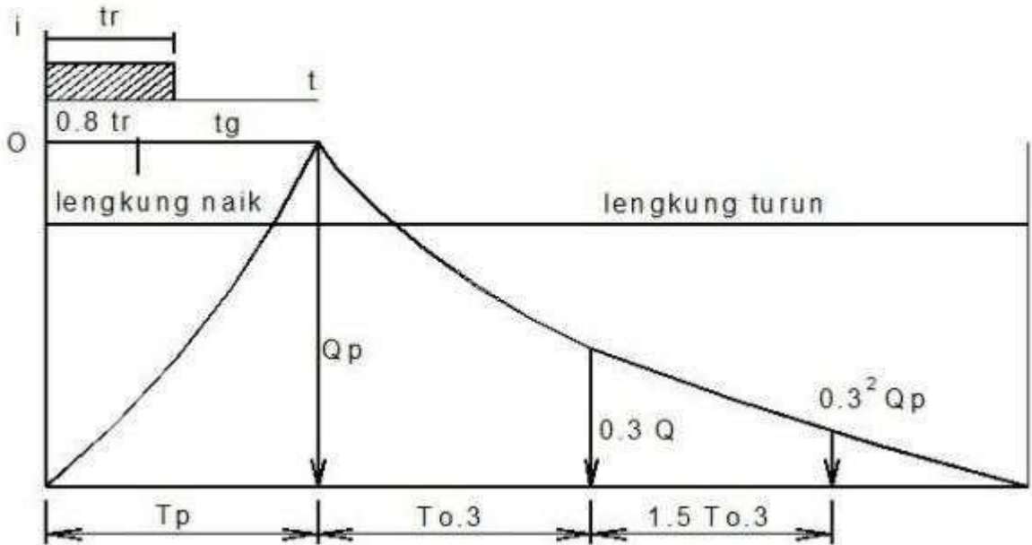
Gambar 2.6. Hidrograf Satuan – Metode Nakayasu
