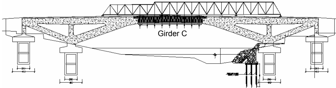
Gambar 14. Tahapan metode pelaksanaan konstruksi
