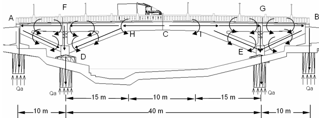
Gambar 6. Mekanisme gaya dalam jembatan dengan sistem penyokong
