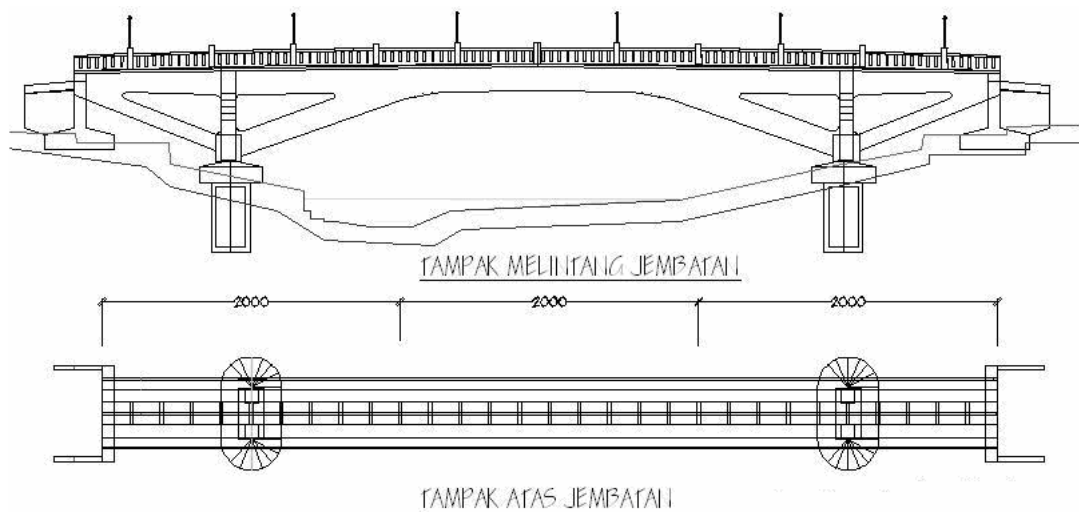
Gambar 5. Tampak melintang dan atas jembatan dengan Sistim Penyokong
