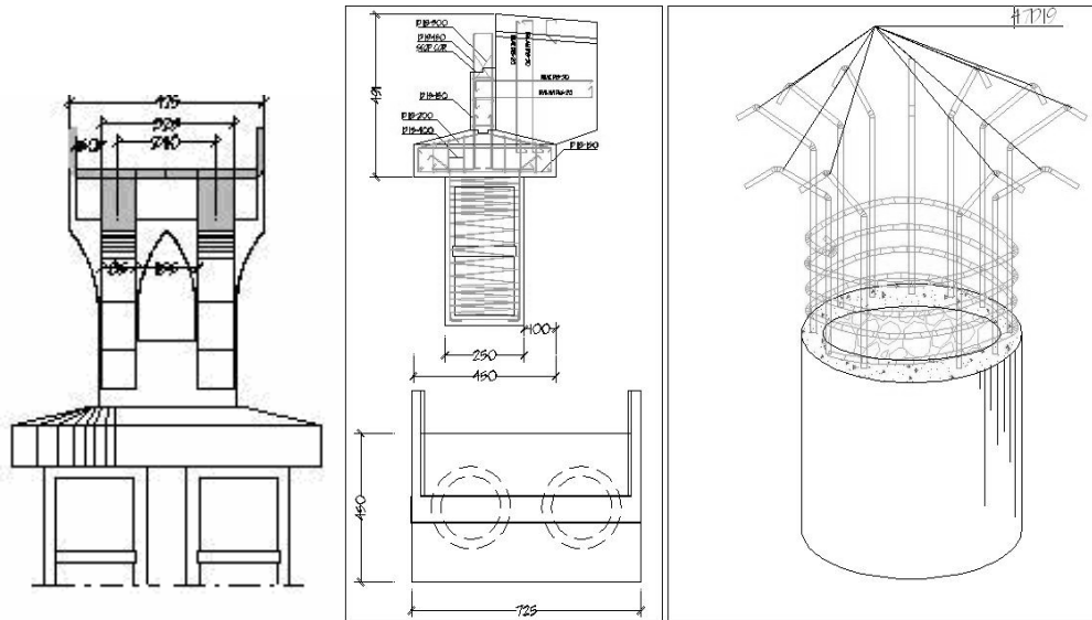
Gambar 13. Pondasi sumuran
