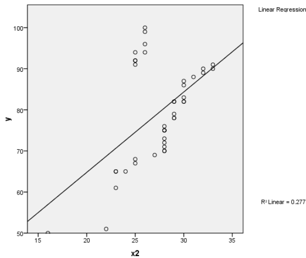
Gambar 4.3. Grafik regresi linear sikap BudAI terhadap hasil tes prestasi geometri analitika 2
