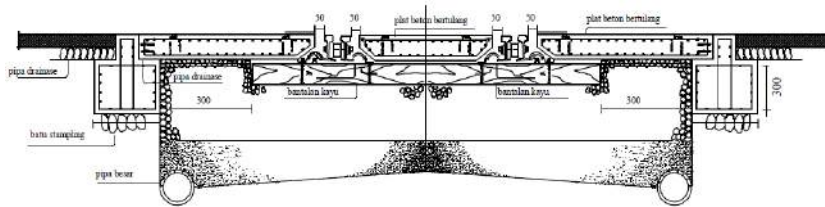
Gambar 1.10. Potongan melintang perlintasan sebidang dengan menggunakan plat beton [9]
